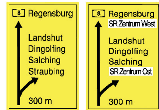
Abstimmung der Vorwegweiser auf das Parkleitsystem: Bestand (links) und Planungsvorschlag (rechts)
